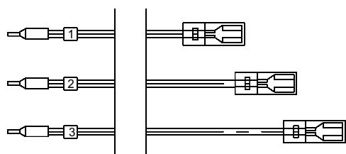
35. Кабель TT - сборка
