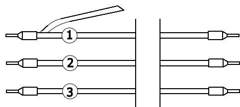
34. Кабель клеммной колодки X1 - сборка (действительно для EK 08K)
