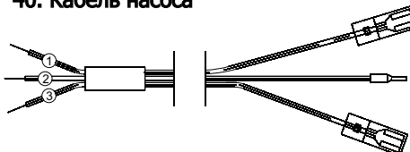
40. Кабель насоса
