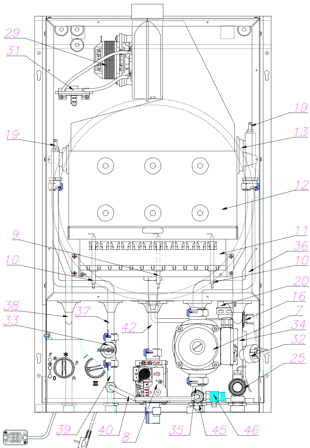
Podstawowe elementy kotła typ GCO-DP-23-57
