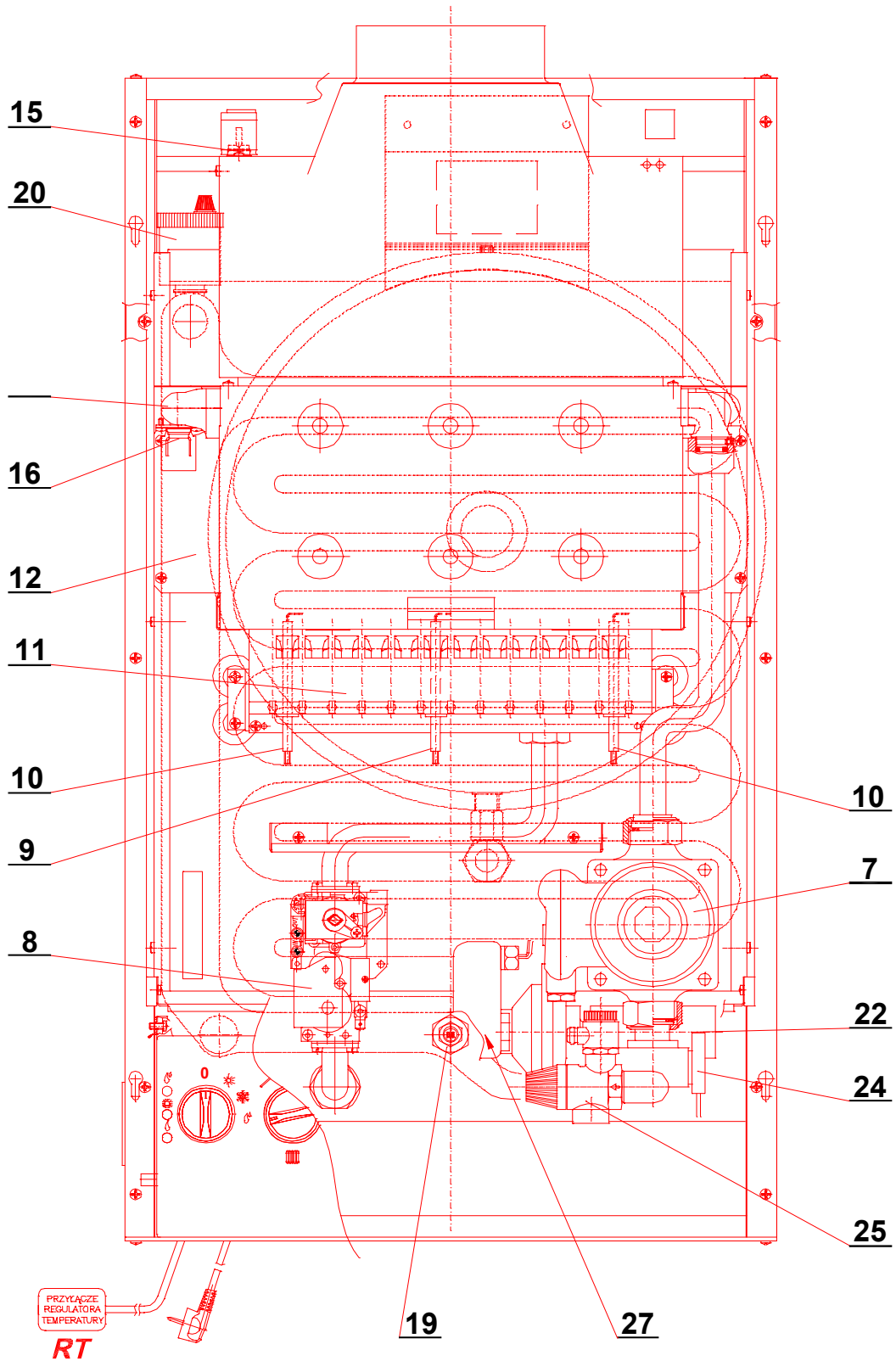
Podstawowe elementy kotła typ GCO-DP-23-37
