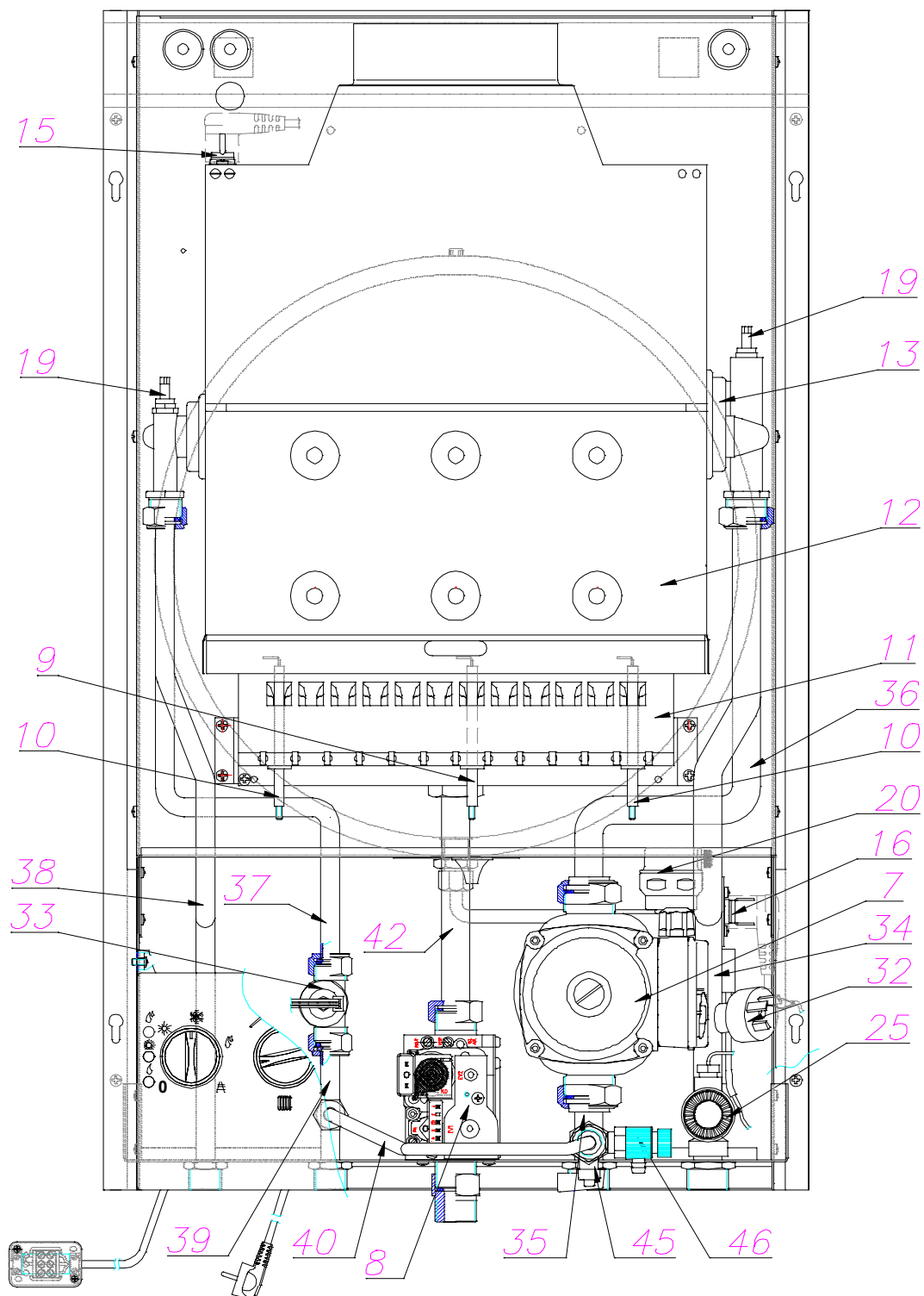
Podstawowe elementy kotła typ GCO-DP-23-47
