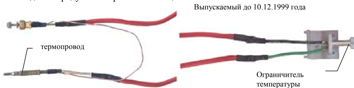
Рис 6 а (370.02.02.00)
