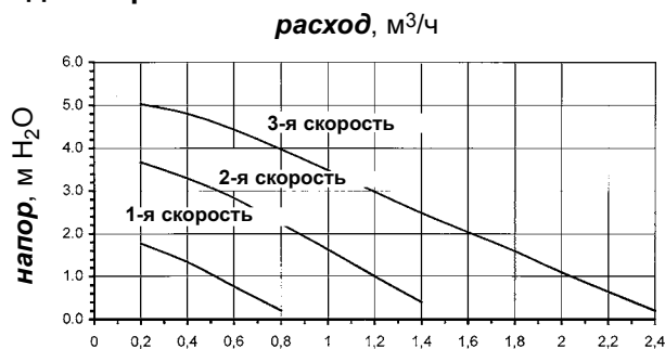
Рис. 12. Кривые расход/напор
